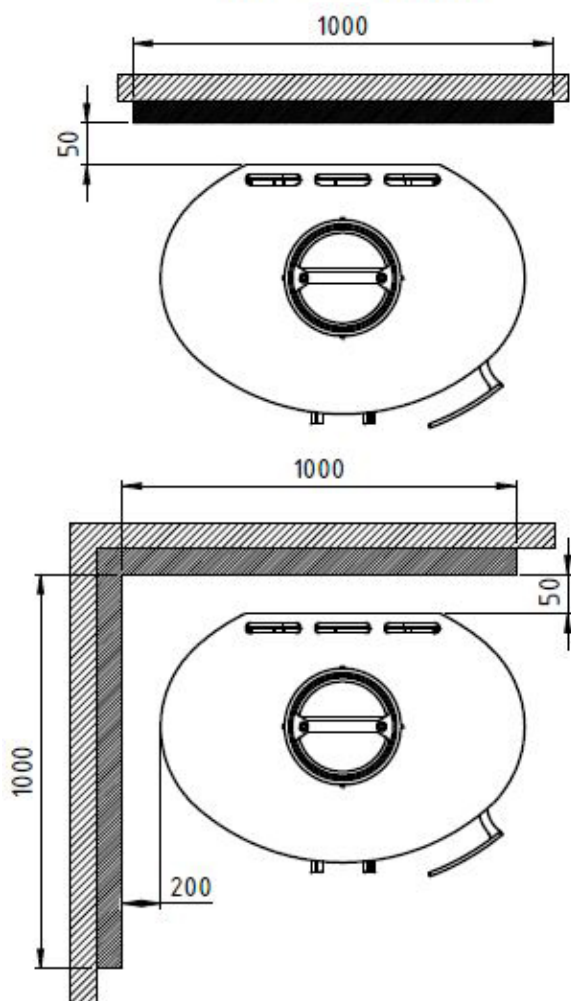
Ild 9 ECO og 11 ECO - uten sideglass
