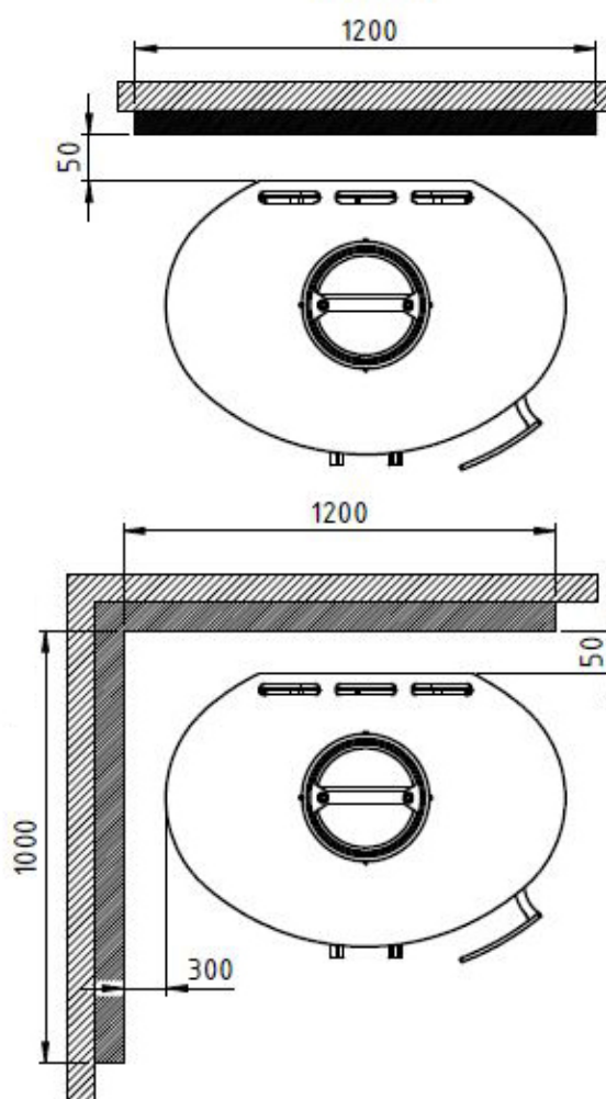
Ild 10 ECO - med sideglass
