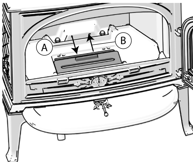
Fig. 13 Askerist
