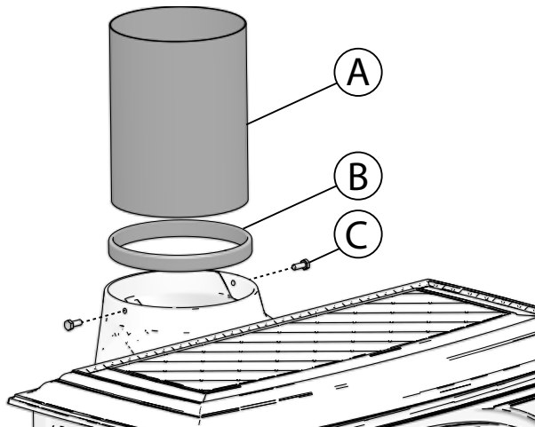
Kuva. 6 Savuputken kiinnittäminen
