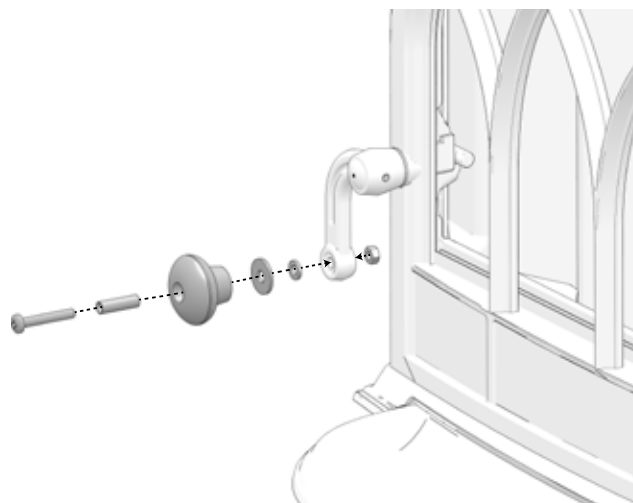
Fig. 3 Dørhåndtagets fastgørelse
