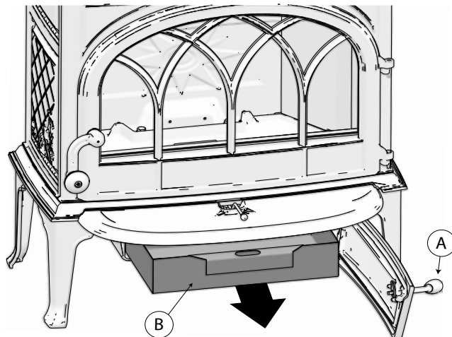
Fig. 14 Askeskuffe
