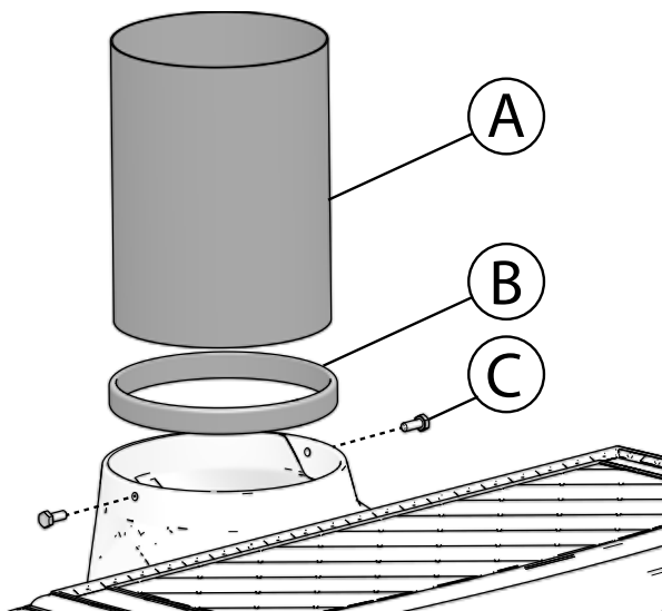
Fig. 6 Montere røgrør
